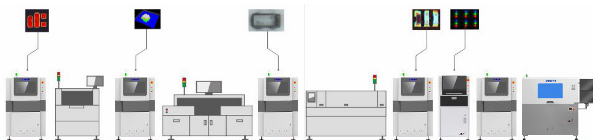
図1: ミニLEDの製造工程における各種光学検査
