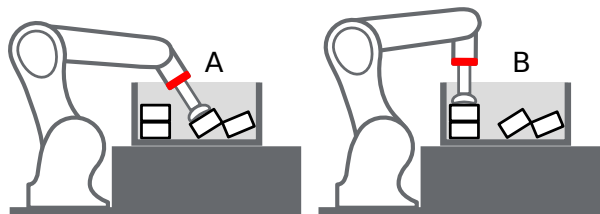
Abb. 6.42: Fall A: Der Griff wird nur als Kollision erkannt, wenn check_flange auf true gesetzt ist, denn der Flansch (rot) befindet sich im Load Carrier. Fall B: Der Griff ist in jedem Fall kollisionsfrei.
