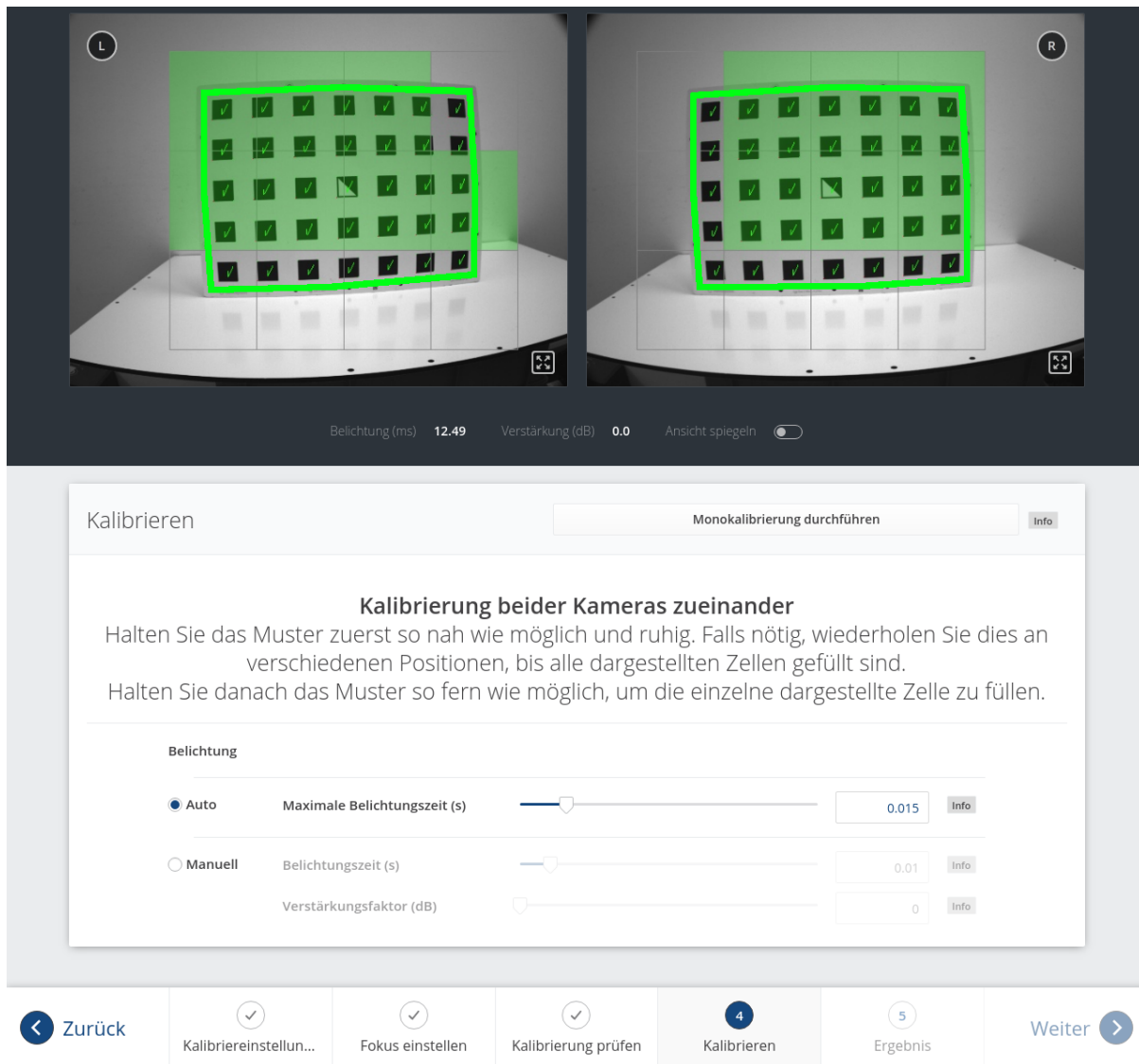
Abb. 6.31: Stereokalibrierung: Das Muster sollte so nah wie möglich gehalten werden, um alle dargestellten Zellen zu füllen.
