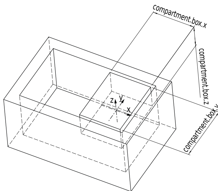
Abb. 6.41: Beispiel für ein Abteil innerhalb eines Load Carriers. Das gezeigte Koordinatensystem das Koordinatensystem des Load Carrier Abteils.
