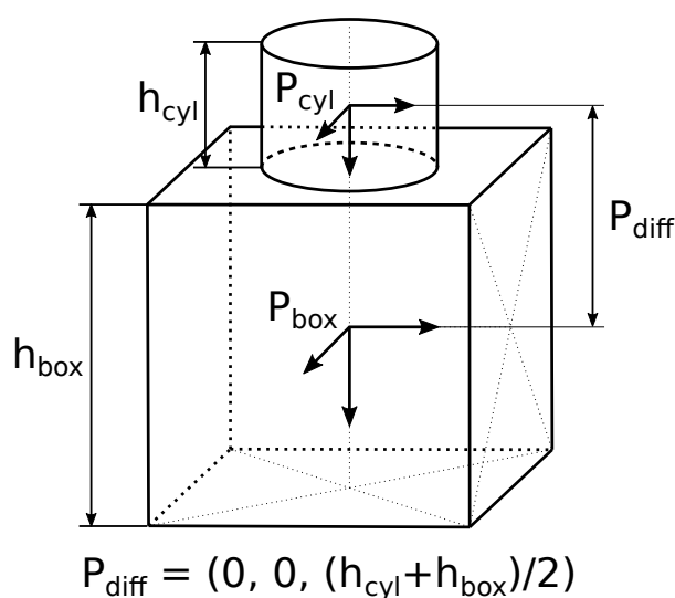
Abb. 6.43: Bezugskoordinatensysteme für das Erstellen von Greifern über die REST-API und die Web GUI
