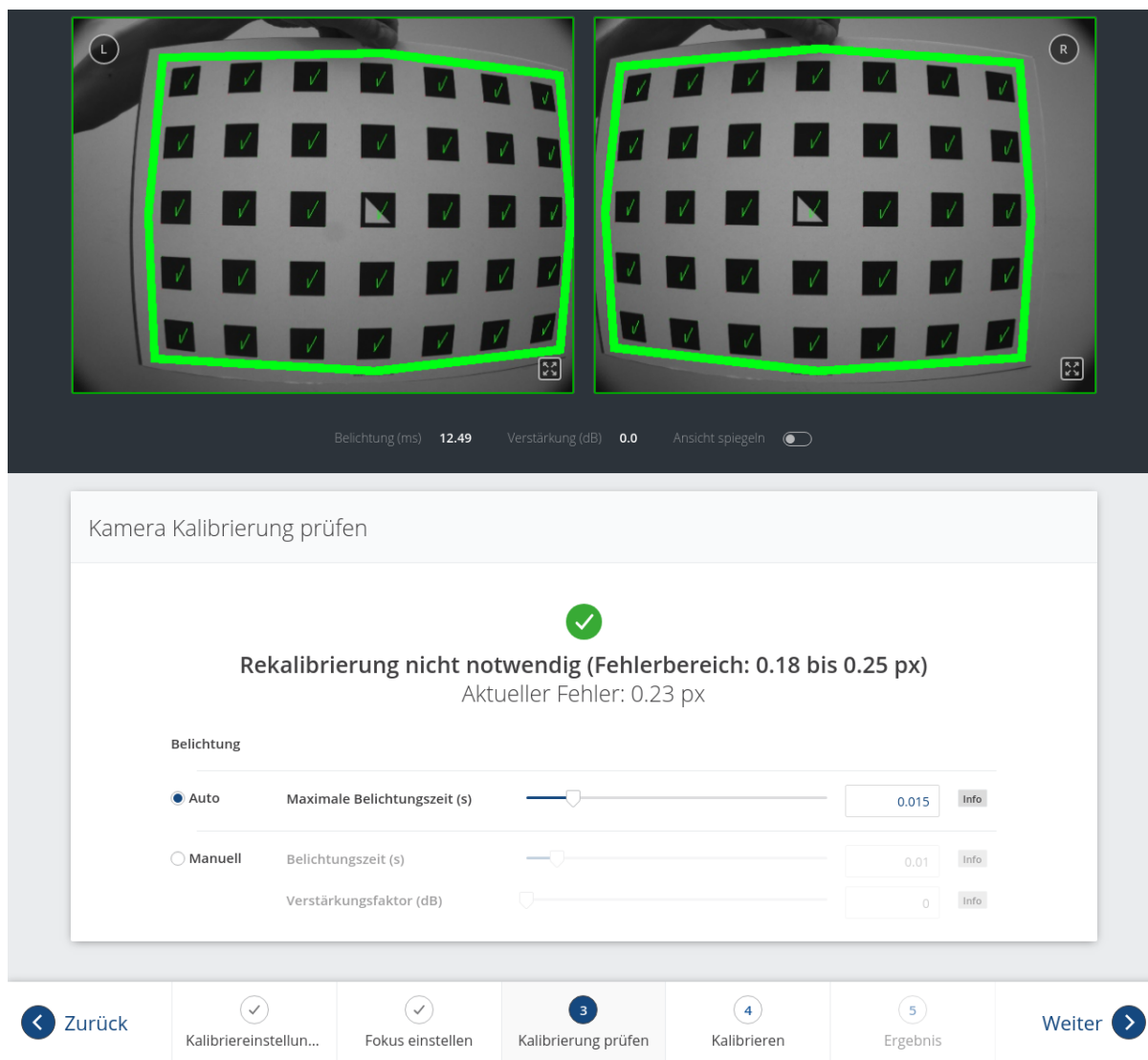
Abb. 6.29: Überprüfung der Kalibrierung
